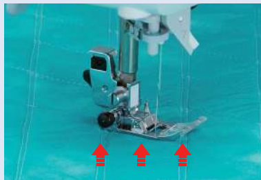
Nähen bei leicht angehobenem Nähfuß.
